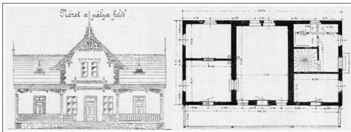
Menyháza-fürdő vasútállomásának tervrajza
